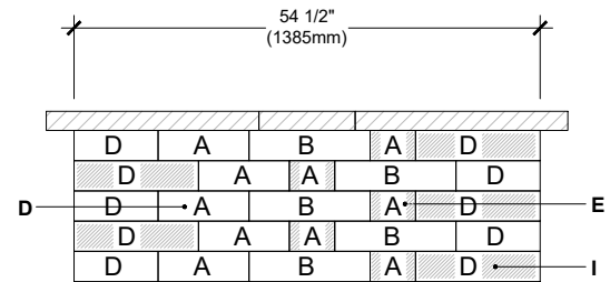
ELEVATION B
