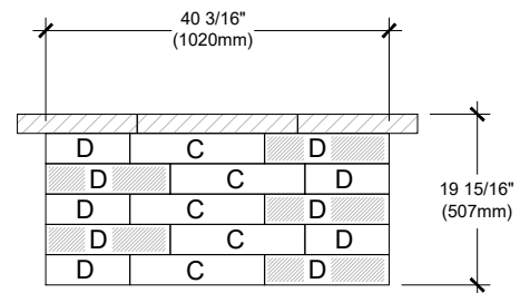
ELEVATION A
