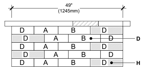
ELEVATION B
