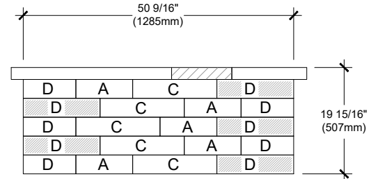
ELEVATION A
