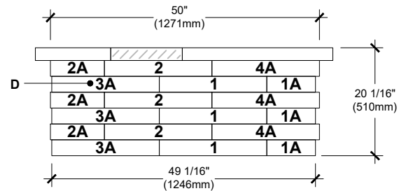
ELEVATION A
