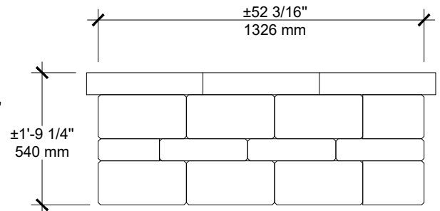
ELEVATION A
