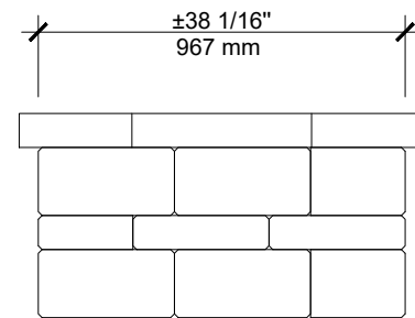
ELEVATION B
