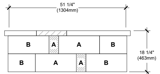
ELEVATION A
