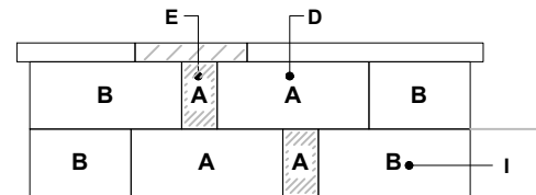
ELEVATION A
