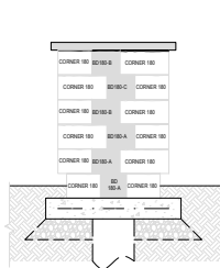
ELEVATION B
