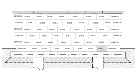
ELEVATION A
