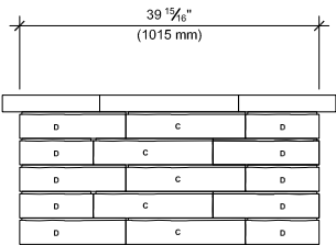
ELEVATION B
