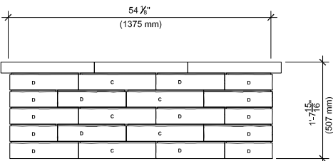
ELEVATION A
