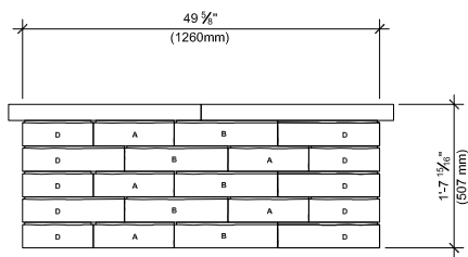
ELEVATION A
